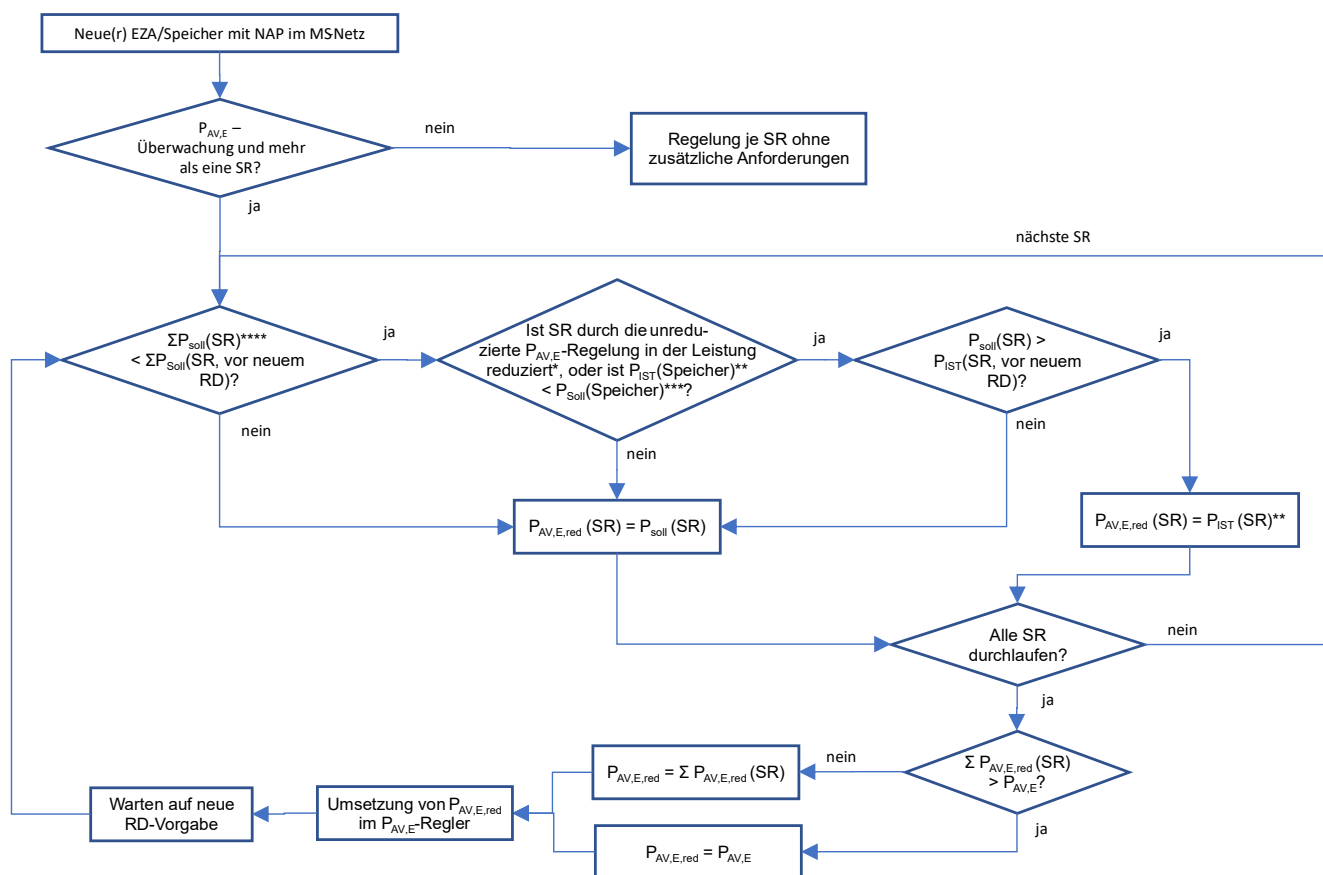
Bild 8.1 Berechnung von P_{AV,E,red} je SR-ID bei einer P_{AV,E} -Überwachung mit mehreren SR-ID's
