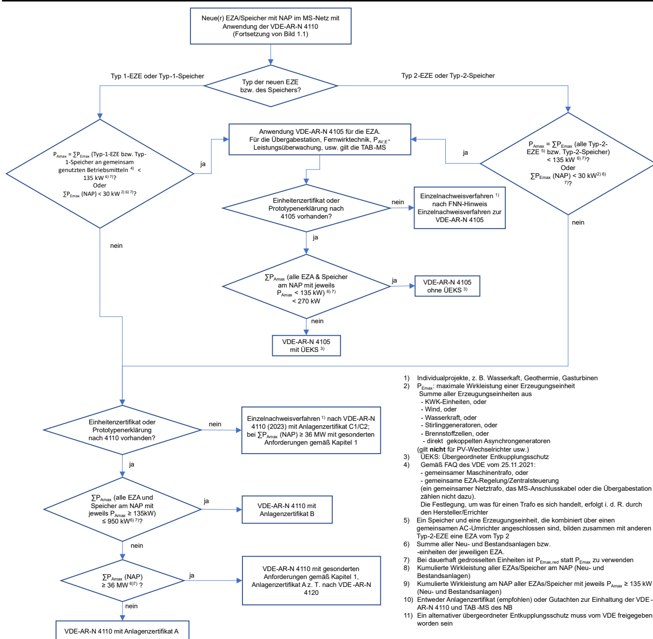
Bild 1.2 Einordnung von Erzeugungsanlagen und/oder Speichern mit Netzanschlusspunkt im Mittelspannungsnetz (ergänzt gemäß der FAQs des VDE/FNN vom 25.11.2021) bzgl. der anzuwendenden Technischen Anschlussregel
