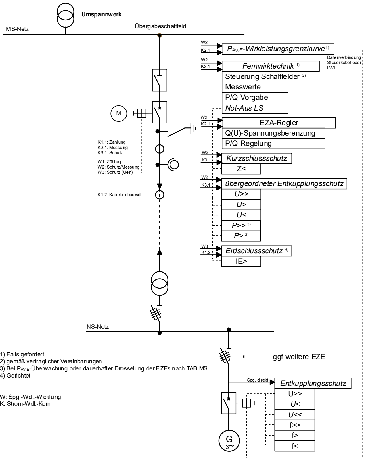
Bild D.15 Einspeisung – Beispiel einer an ein Umspannwerk mittelspannungsseitig angeschlossenen Erzeugungsanlagen mit Leistungsschalter und Erzeugungseinheit ohne Inselbetriebsmöglichkeit
