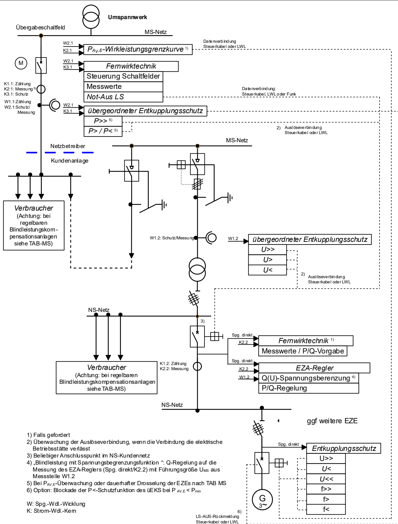
Bild D.17 Mischanlage – Beispiel einer an ein Umspannwerk mittelspannungsseitig angeschlossenen Kundenanlage mit Bezug und Erzeugungsanlage mit Leistungsschalter und einer Erzeugungseinheit ohne Inselbetriebsmöglichkeit
